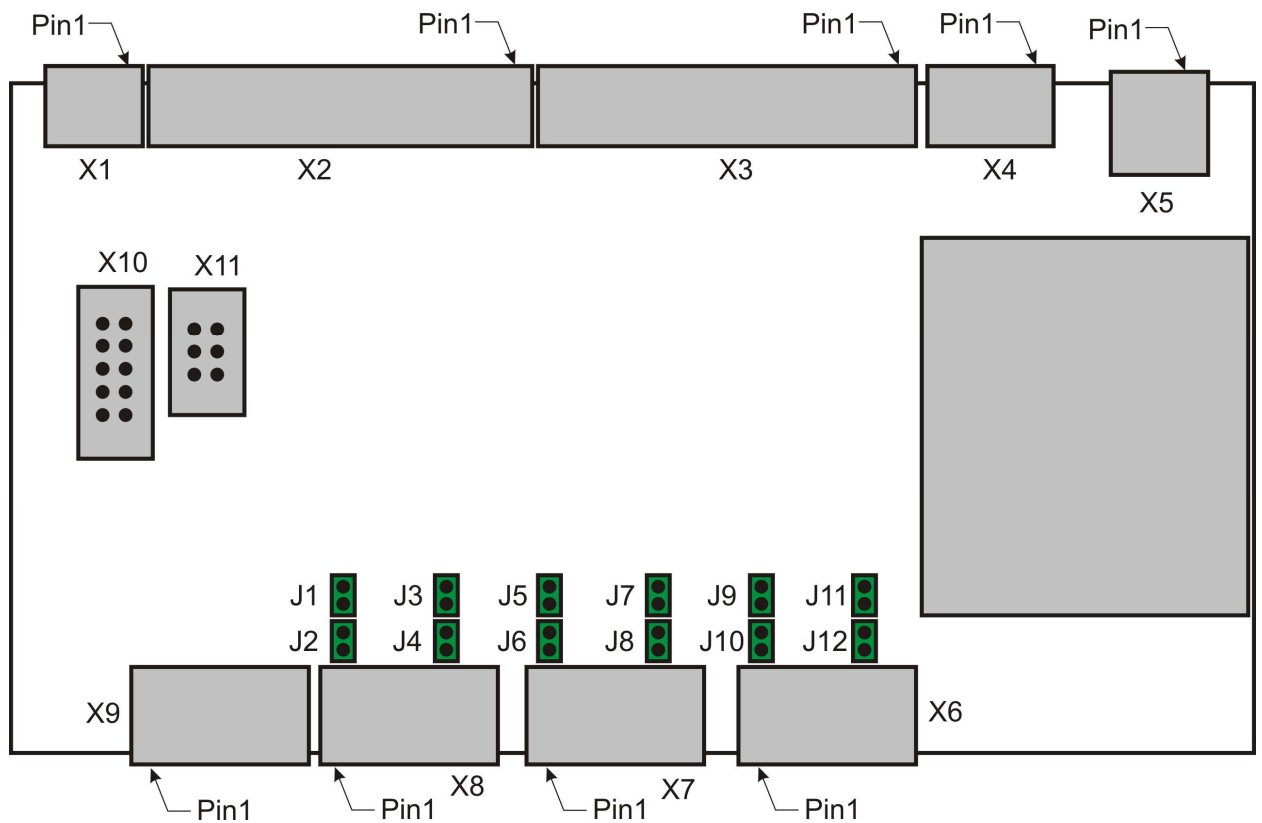
Рисунок 25 - Расположение джамперов на печатной плате
