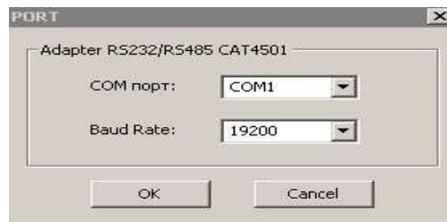
Рисунок 10 - Настройка интерфейса с модулями
