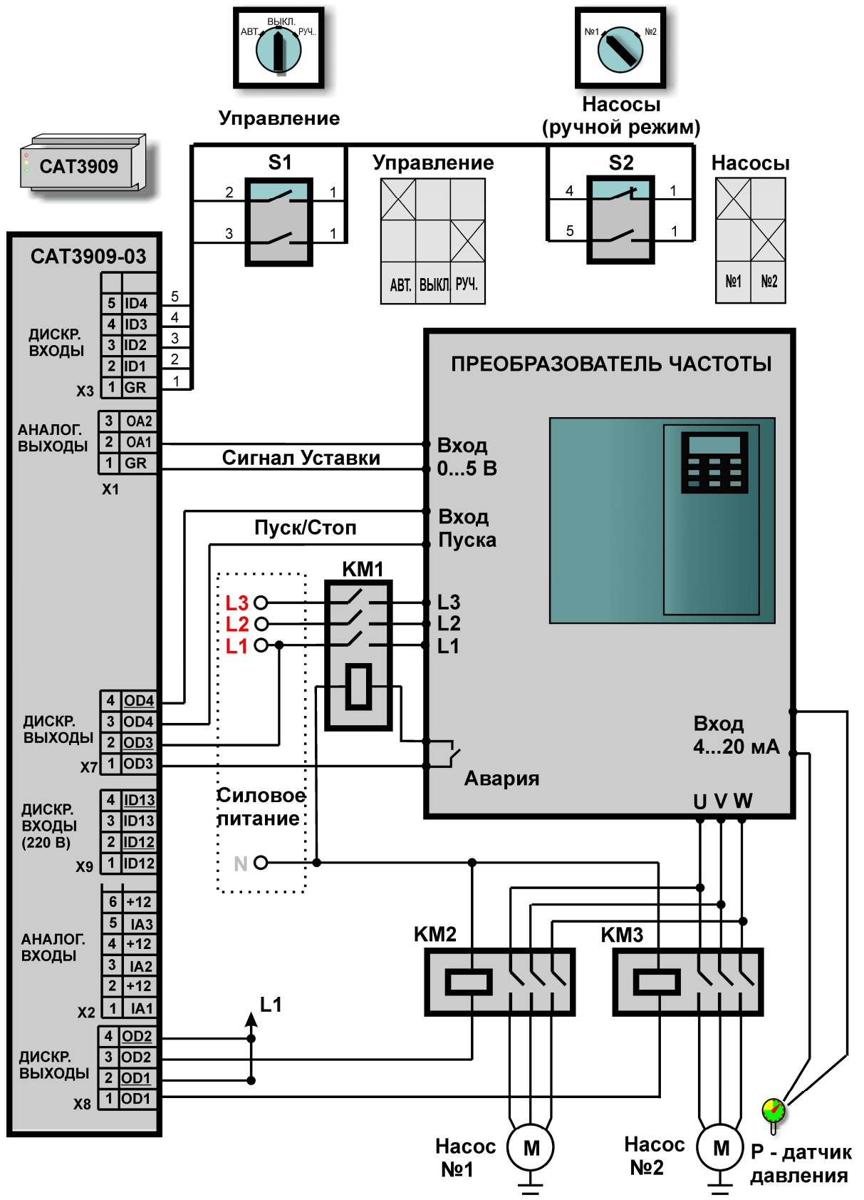
Рисунок 27 - Вариант подключения модуля
