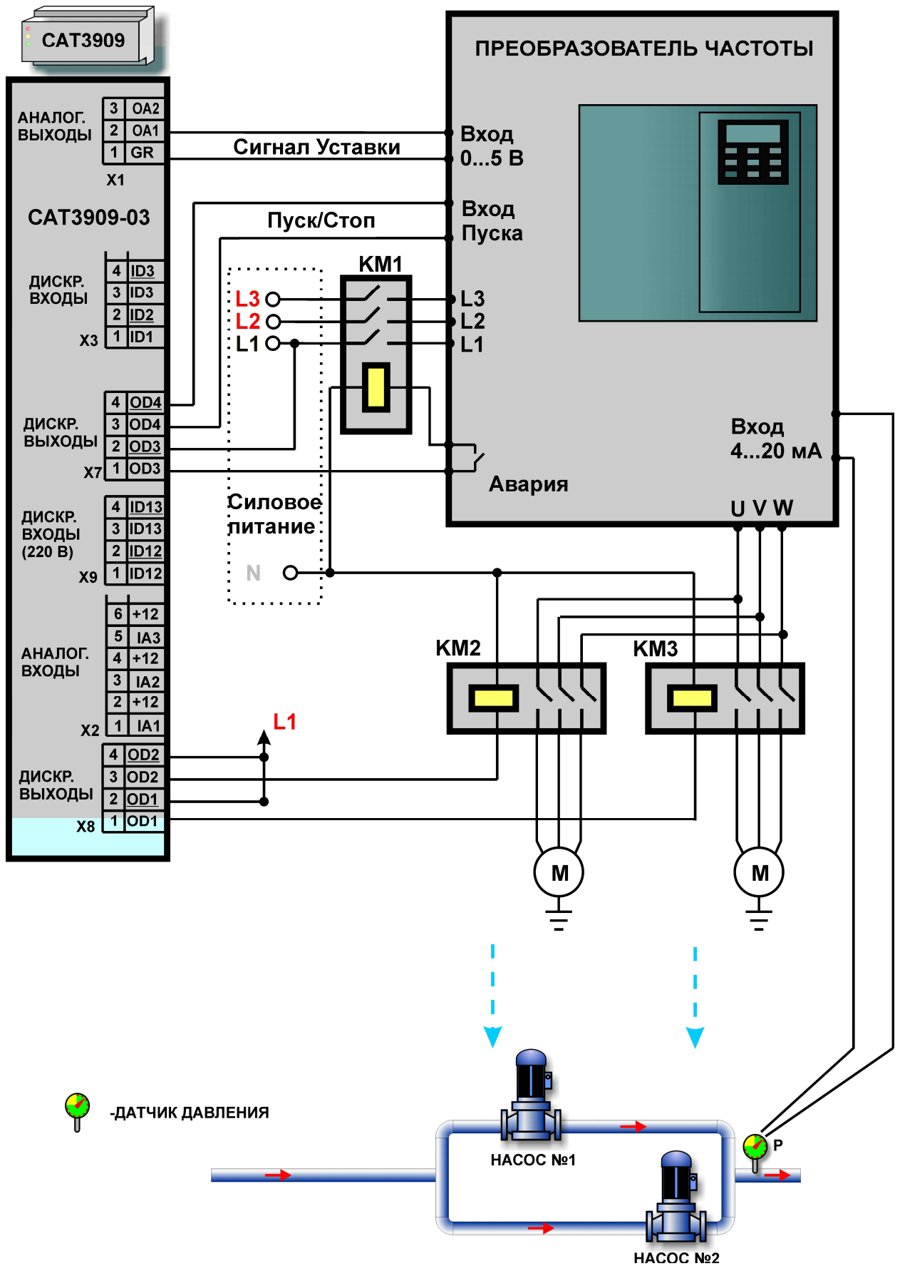
Рисунок 5 - Электрическая схема подключения КАТ3909-03 (типовая)
