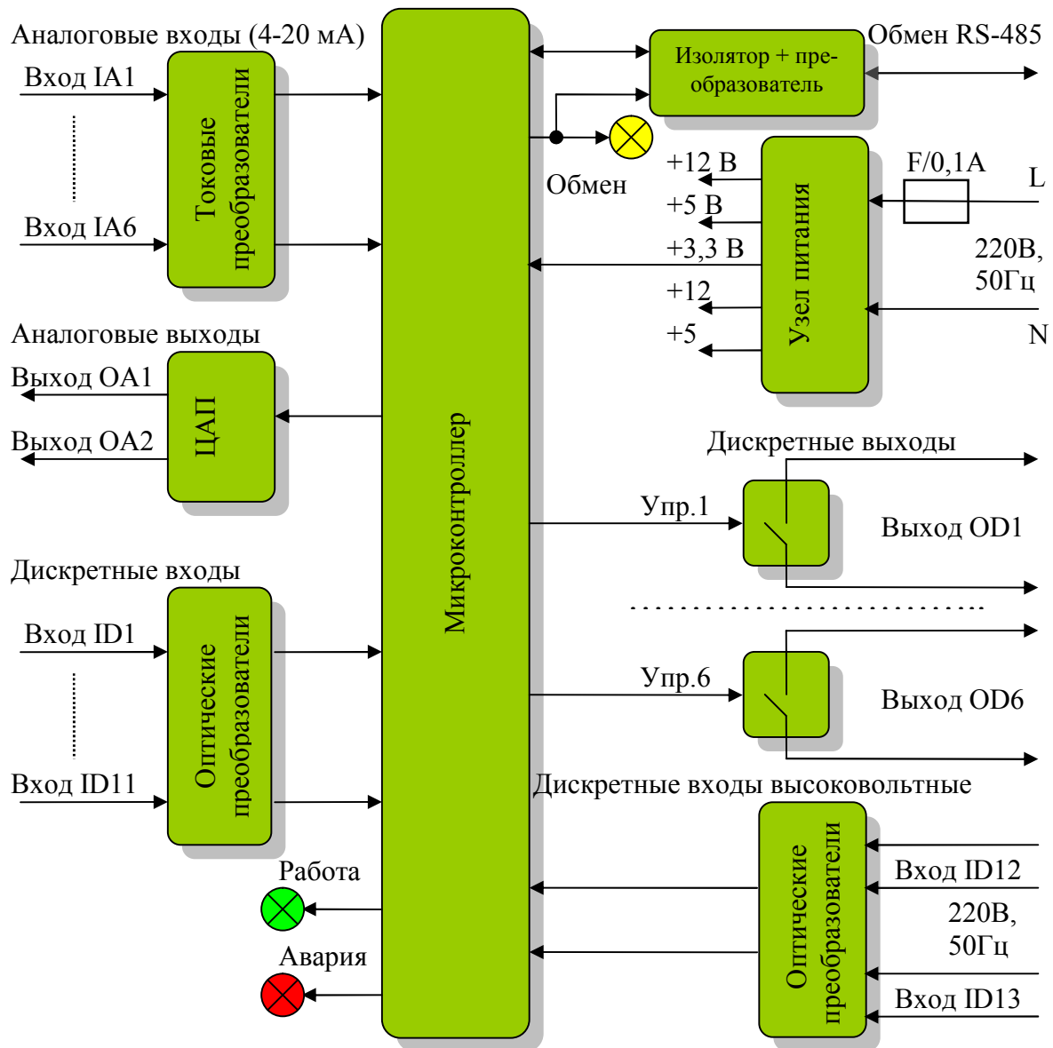
Рисунок 2 - Структурная схема САТ3909-03
