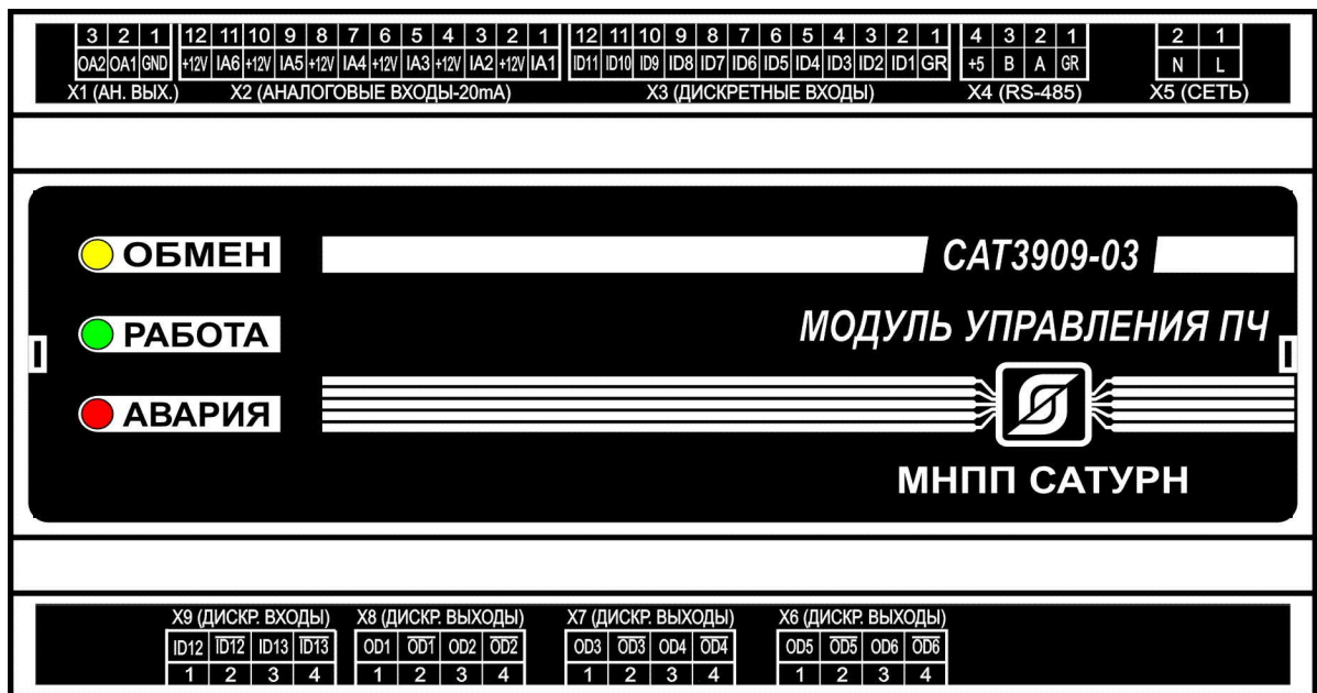
Рисунок 1- Внешний вид модуля САТ3909-03
