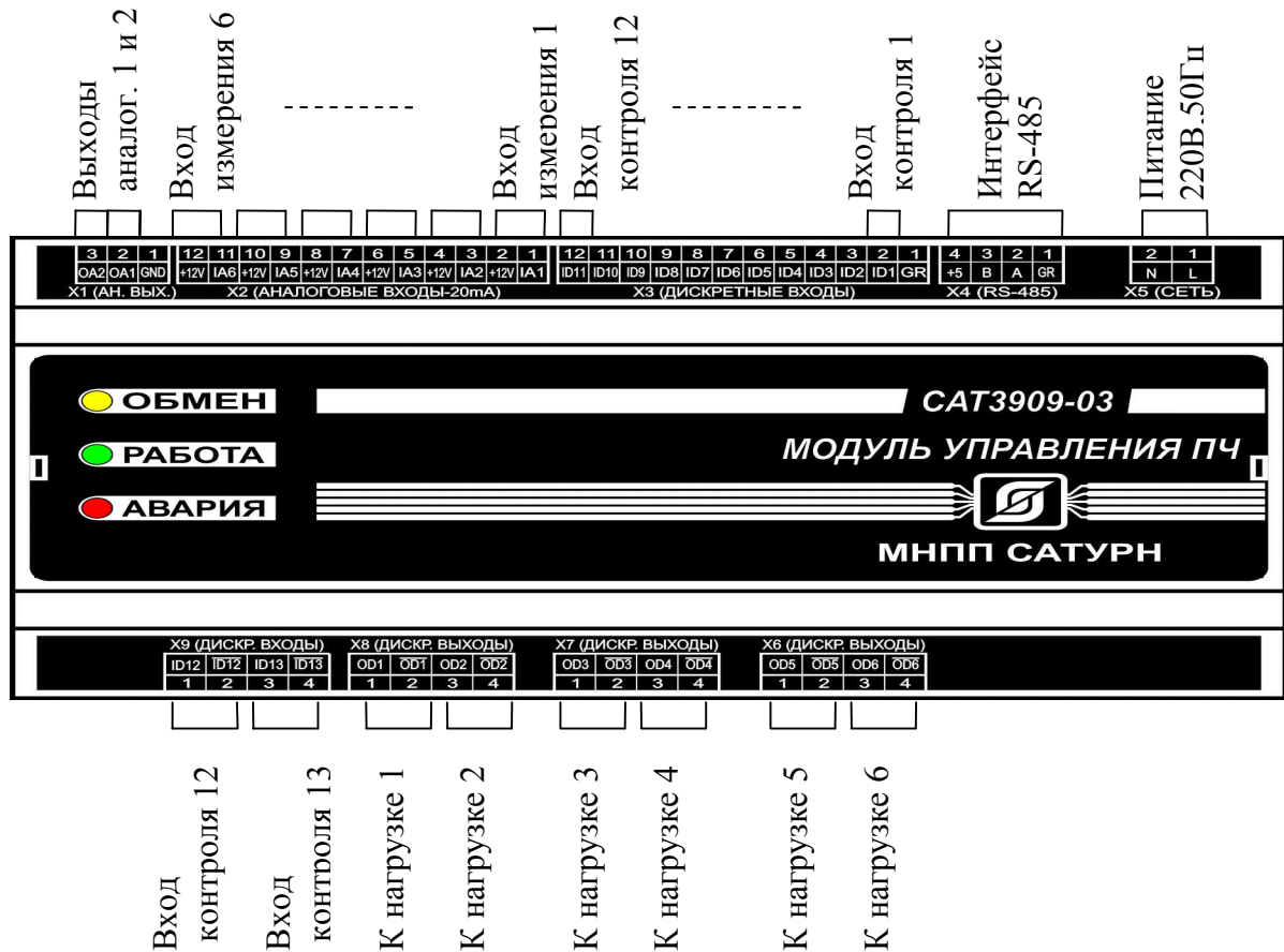
Рисунок 4 - Расположение разъёмов на модуле САТ3909-03
